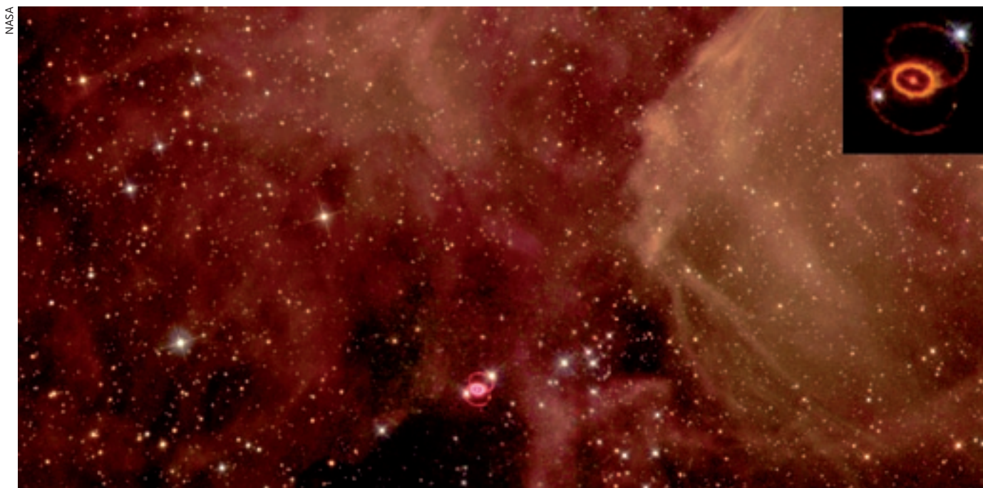
Imagen de la Supernova 1987A tomada desde el telescopio espacial Hubble. Los neutrinos provocan la expulsión de buena parte de la masa de la estrella al medio interestelar.
